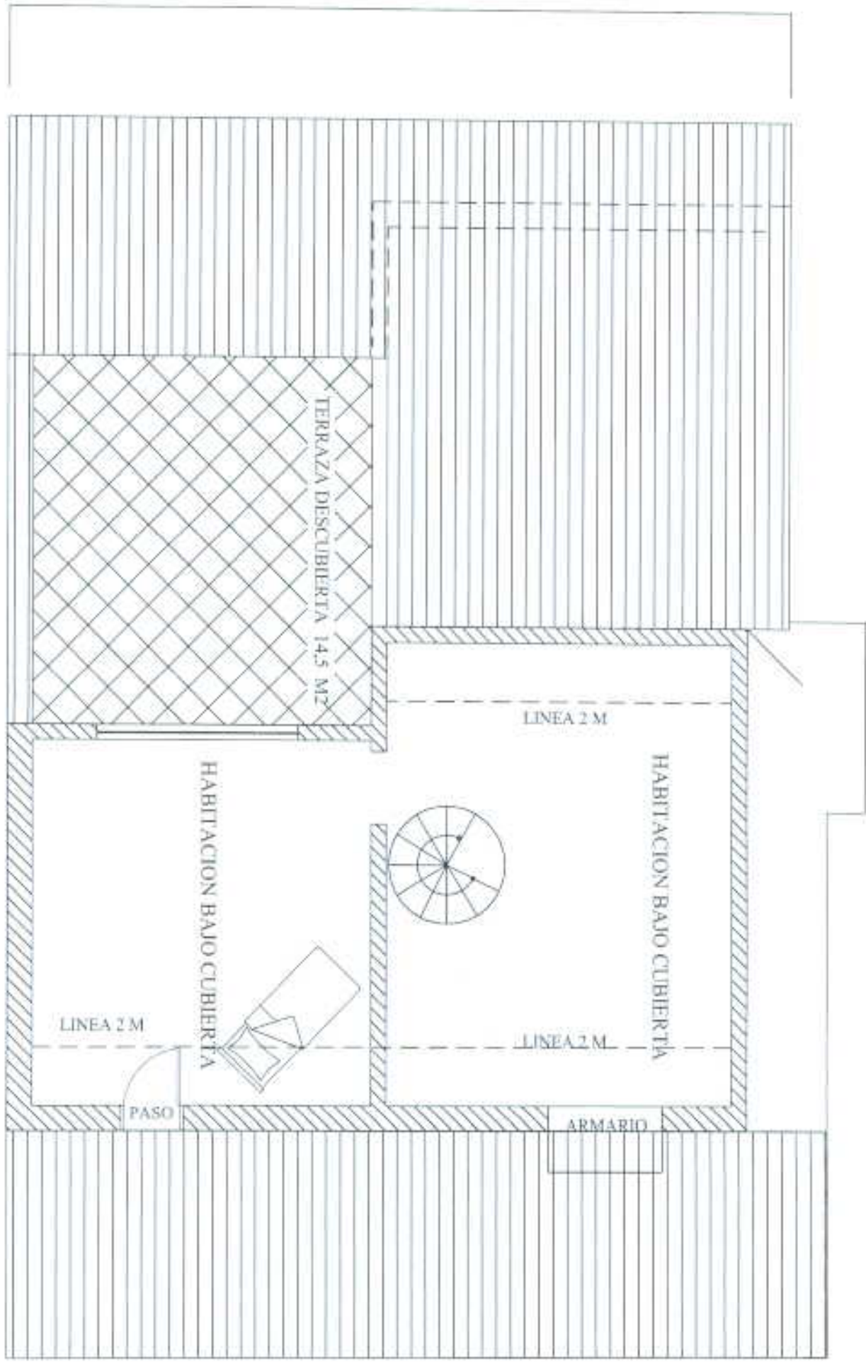
PLANTA 1ª E.1:50
